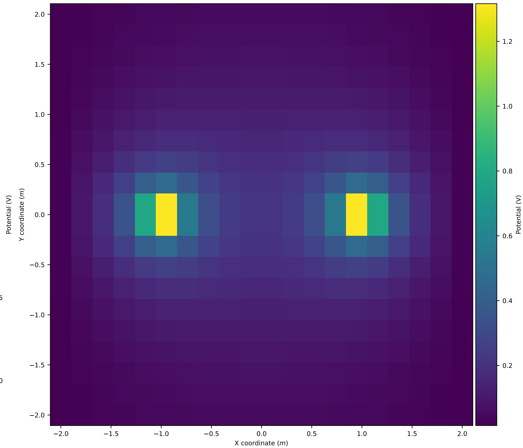
4 Electrodes
